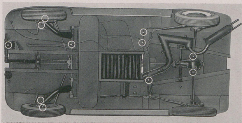
Die Schmierstellen
