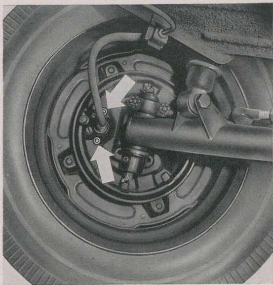
Nachstellen der Öldruckbremse
