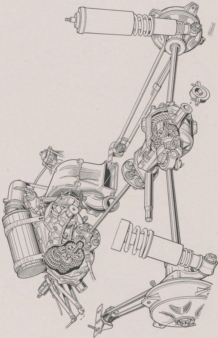
Hinterachse mit Antriebsaggregat
