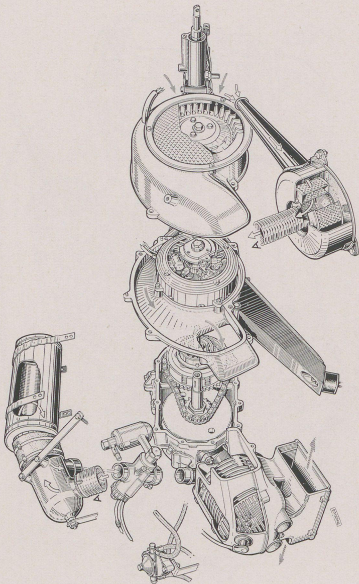
Motor, Gebläseseite mit Anlaß-Lichtmaschine und Ansaugluftführung
